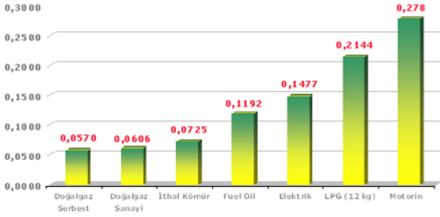
Ekim 2006 Sanayi Yakıt Karşılaştırması (YTL/1000 kcal)
