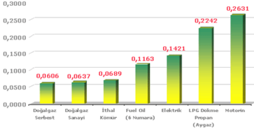
Aralık 2007 Sanayi Yakıt Karşılaştırması (YTL/1000 kcal)
